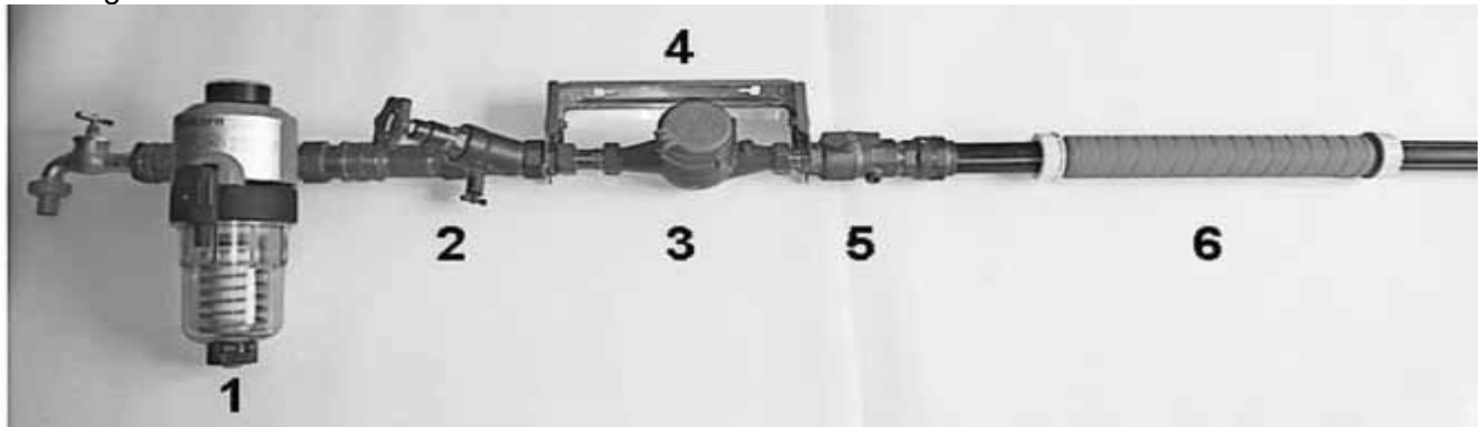
Skizze (Foto mit Beschriftung/Erläuterung) Wasserzähleranlage
