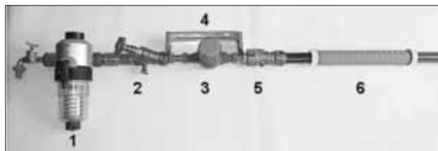
Skizze (Foto mit Beschriftung/Erläuterung) Wasserzähleranlage
