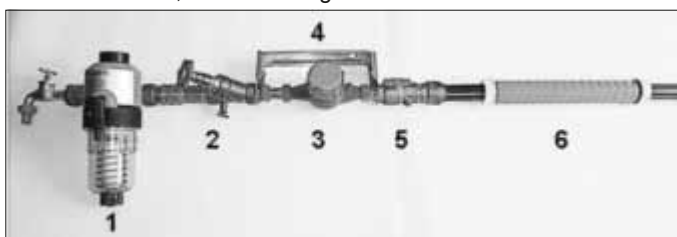
Skizze (Foto mit Beschriftung/ Erläuterung) Wasserzähleranlage
