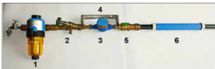
Skizze (Foto mit Beschriftung/Erläuterung) Wasserzähleranlage
