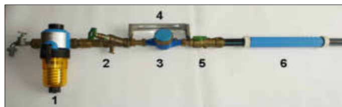
Skizze (Foto mit Beschriftung/Erläuterung) Wasserzähleranlage
