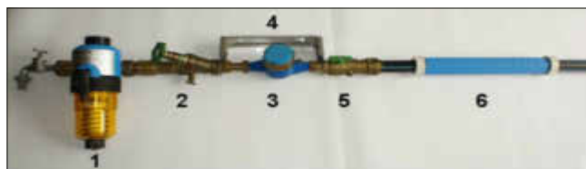
Skizze (Foto mit Beschriftung/Erläuterung) Wasserzähleranlage
