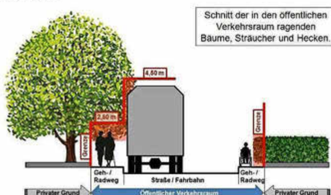
Lichttraumprofil:
